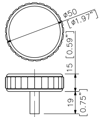
Knob bolt
